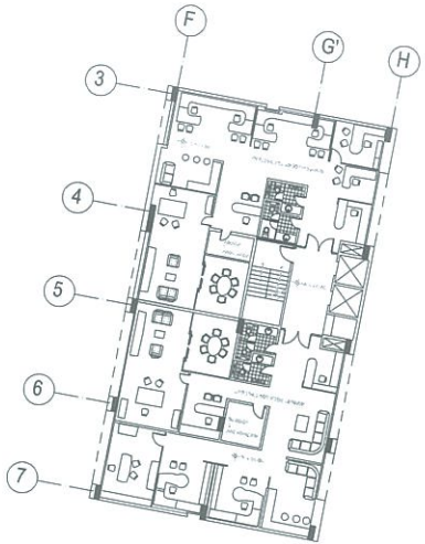
PLANTA+14.90 ESC 1:200
