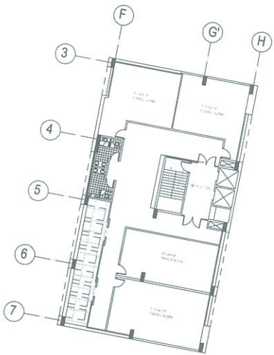
PLANTA+17.90 ESC 1:200
