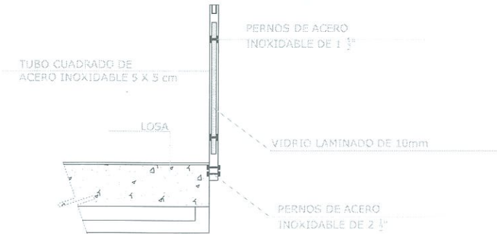
CORTE PASAMANO A-A' ESC 1:10
