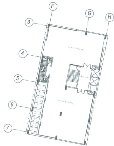
PLANTA+17.90 ESC 1:200
