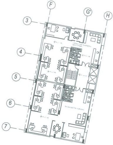
PLANTA+11.90 ESC 1:200
