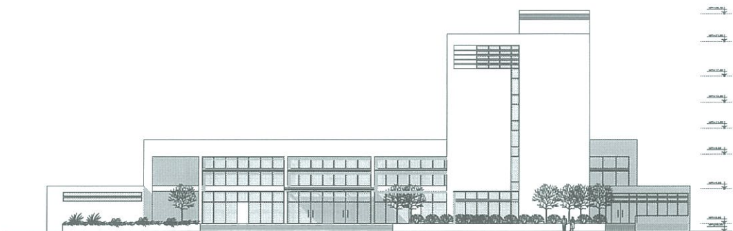
FACHADA CALLE UNP ESC 1:200
