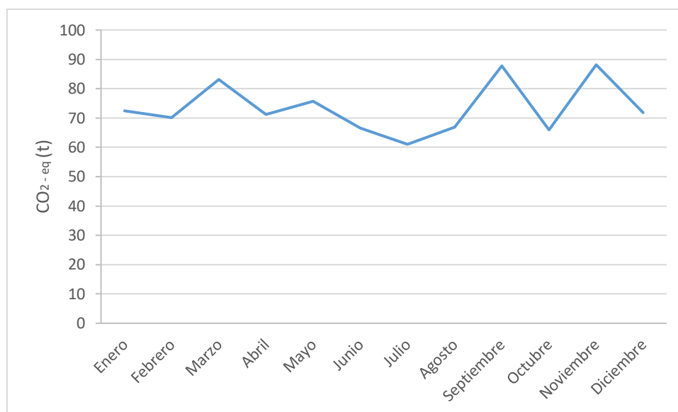
Figura 2. Emisión mensual de CO 2 – eq
