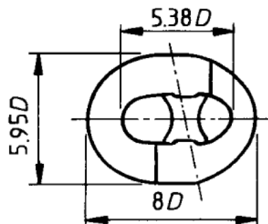
Figura 111. Argolla de conexión tipo de pera (Almazán Gárate, Palomino Monzón, Paramio Cabrera, & Espinosa Goded).
