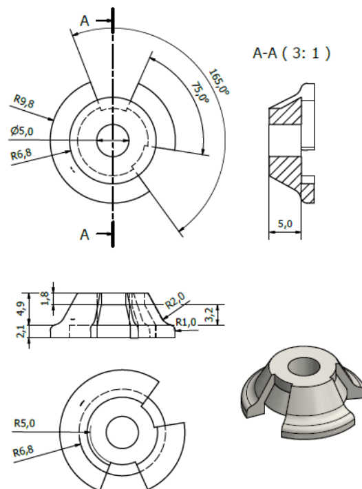
Figura 14. Dimensiones del Flange
