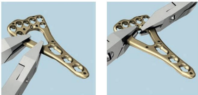
Figura 15: doblar las placas utilizando alicates planos
