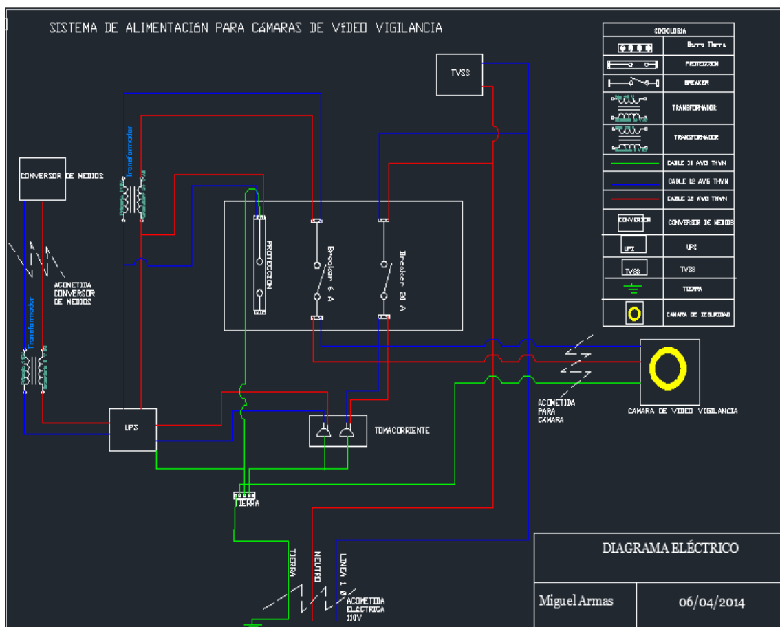
Figura 8 Diseño Plano Eléctrico AutoCAD.
