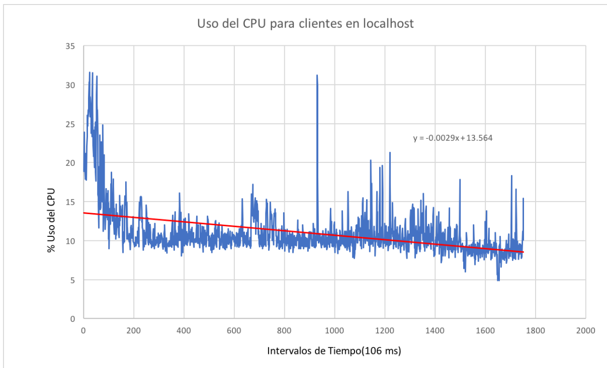
Figura 6: Uso del CPU para clientes en localhost
