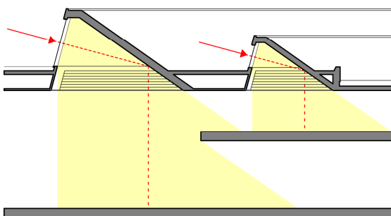
DIAGRAMA ILUMINACION CORTE ILUMINACION BIBLIOTECA VIRGILIO BARCO VARGAS
