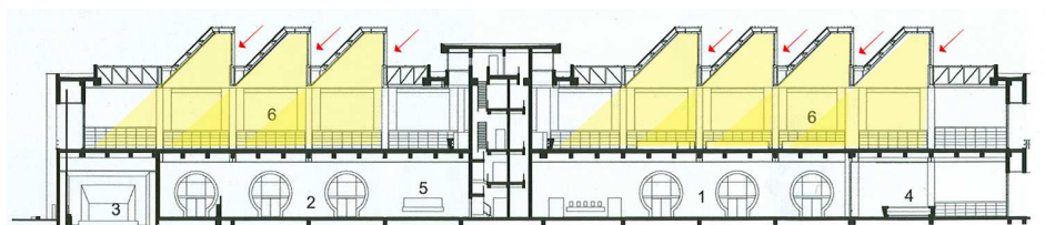
INGRESO DE LUZ POR LA CUBIERTA
