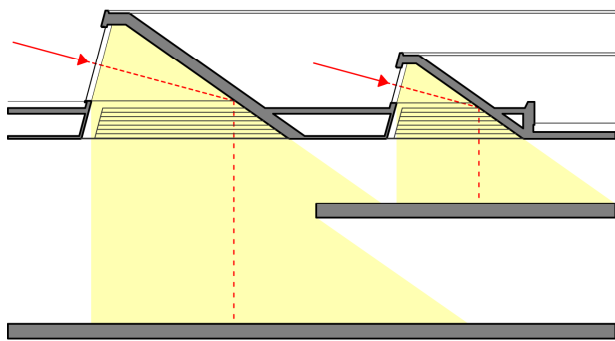
DIAGRAMA ILUMINACION CORTE
